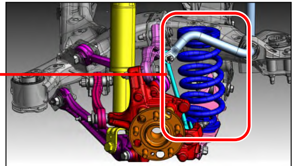
リヤ緩衝装置
